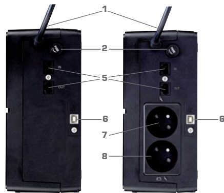
Face arrière modèle 500 VA
